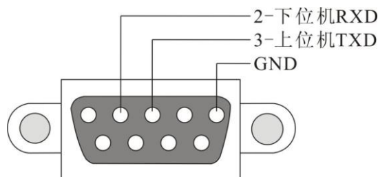
图 8-2-1 通信接口
