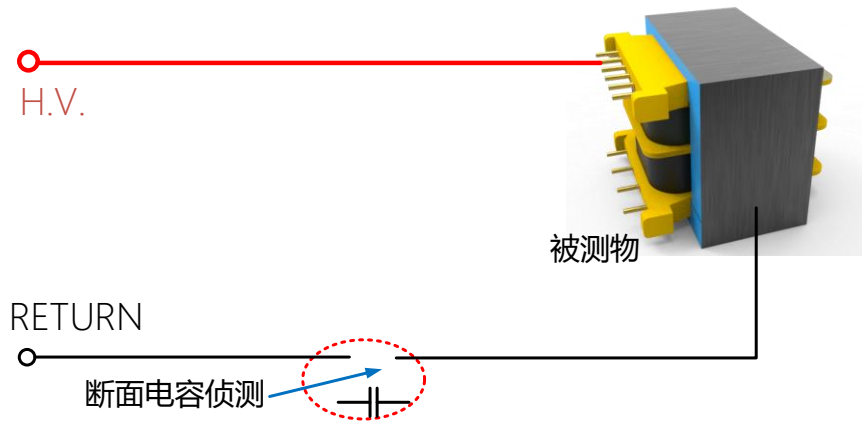
图 5-5-8 开路侦测测试基本原理
