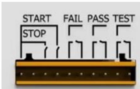
图 6-1-1 PLC 接口插座（公）
