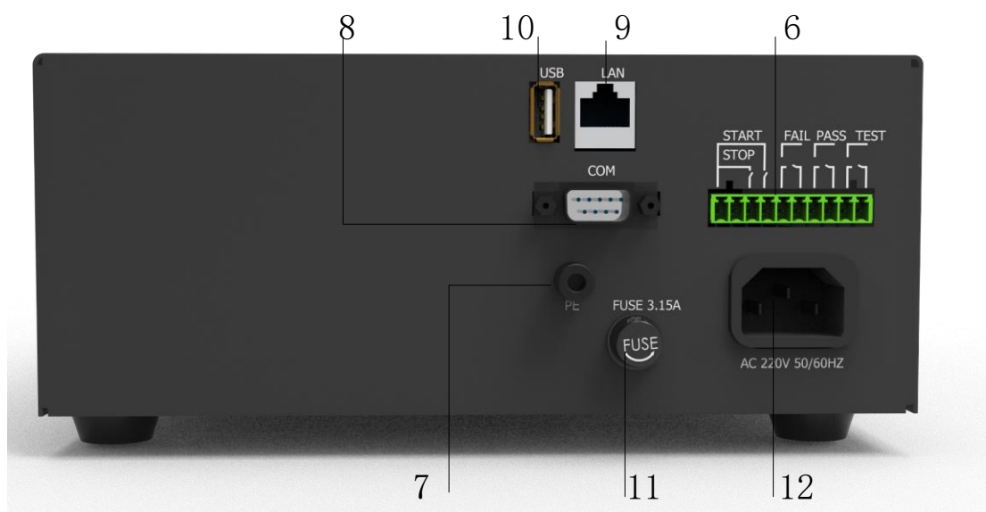
图 4-3-1 后面板
