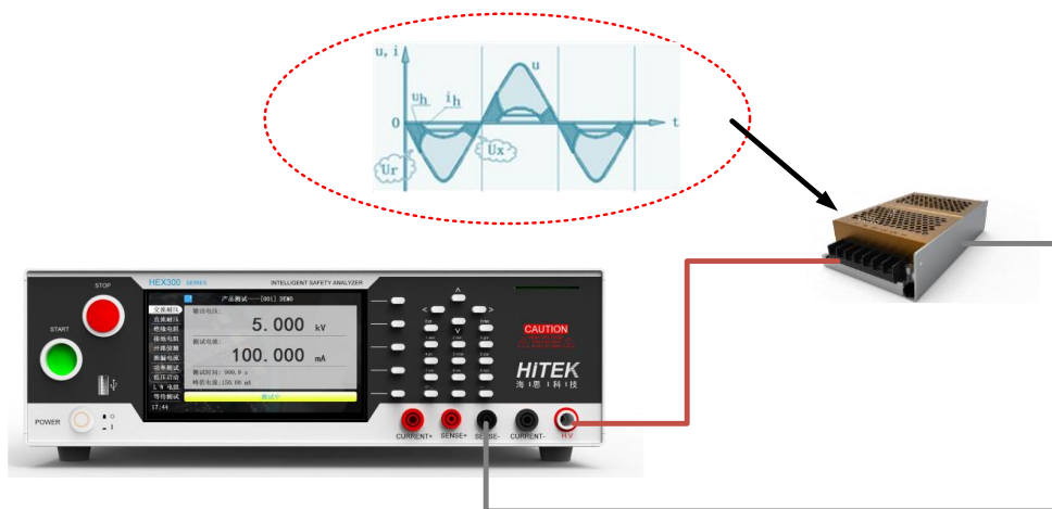
图 3-1-3 电弧侦测
