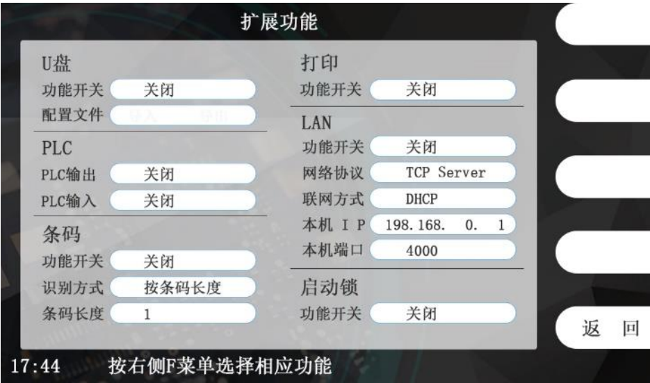
图 5-7-1 扩展功能界面
