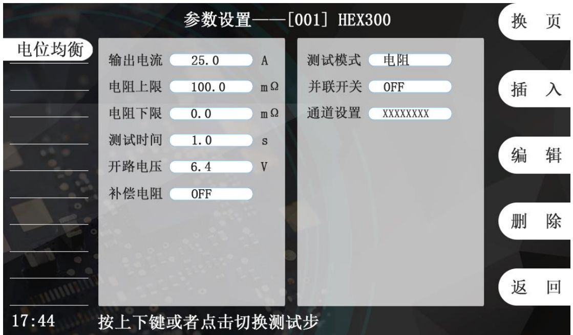
5-5-6 电位均衡设置界面
