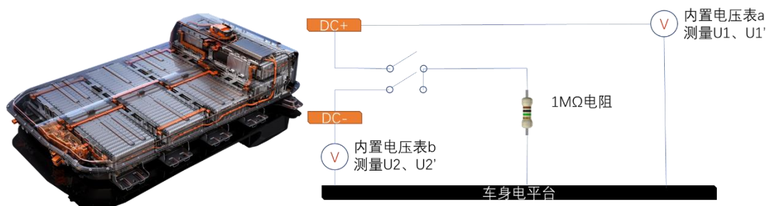
图 5-1-3 电池包绝缘测试接线示意图
