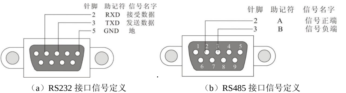
图 6-7-1 通信接口定义
