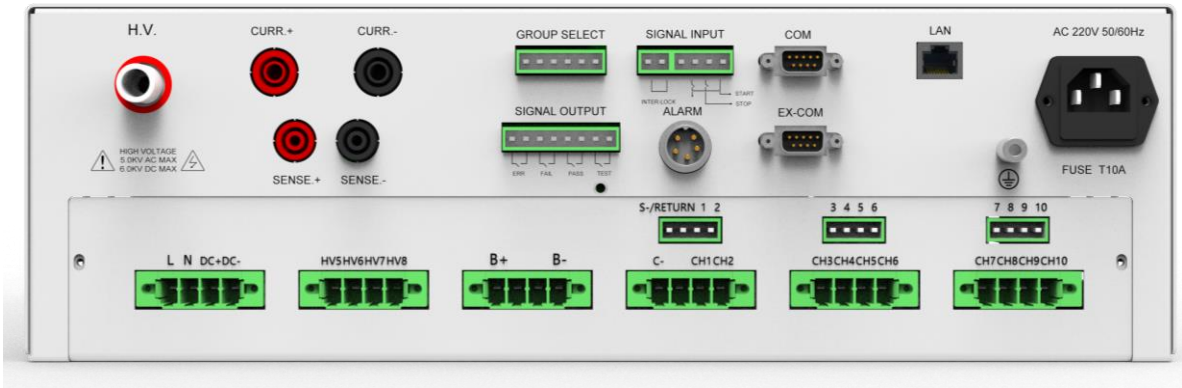
图 3-1-6 后面板
