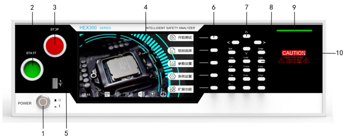
图 4-2-1 HEX350 系列前面板
