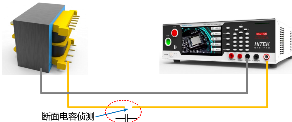
图 3-1-2 断面电容侦测
