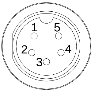
图 6-1-1 报警灯口插座（公）
