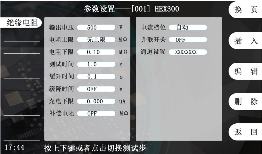
图 5-5-4 绝缘电阻设置界面
