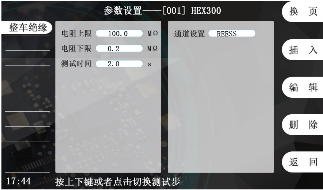
图 5-5-6 整车绝缘设置界面
