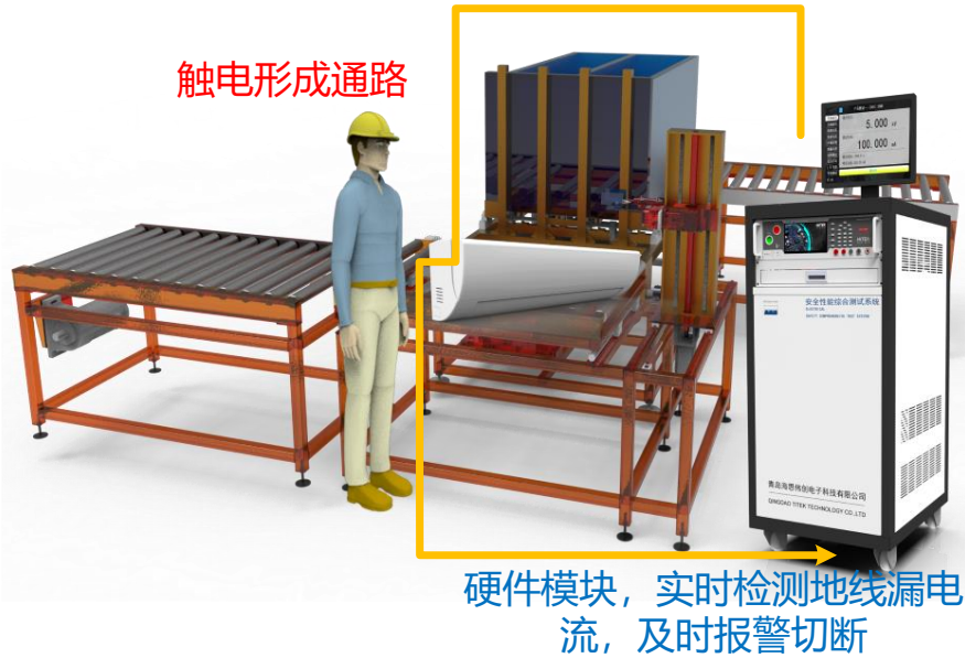
图 3-1-1 漏电快速断电保护原理
