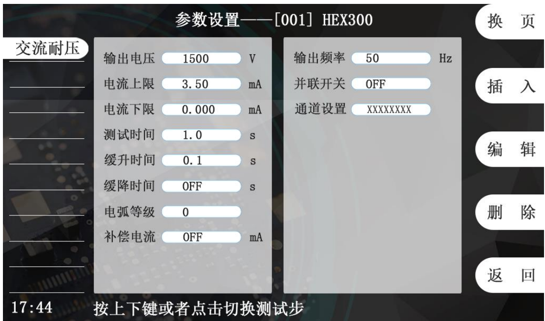
图 5-5-1 测试组设置界面
