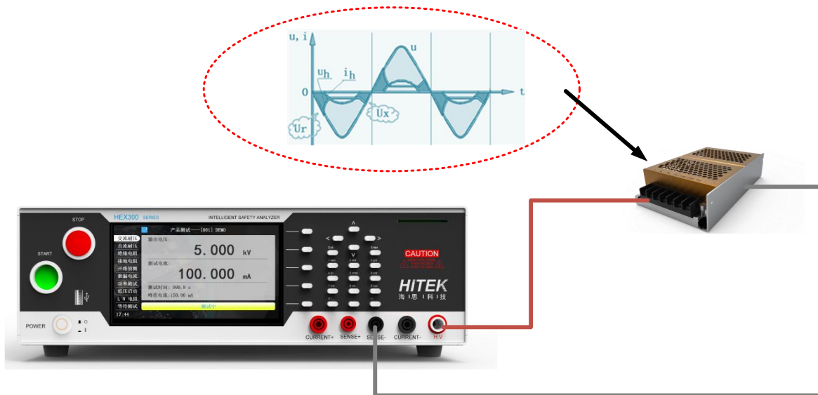
图 3-1-3 电弧侦测
