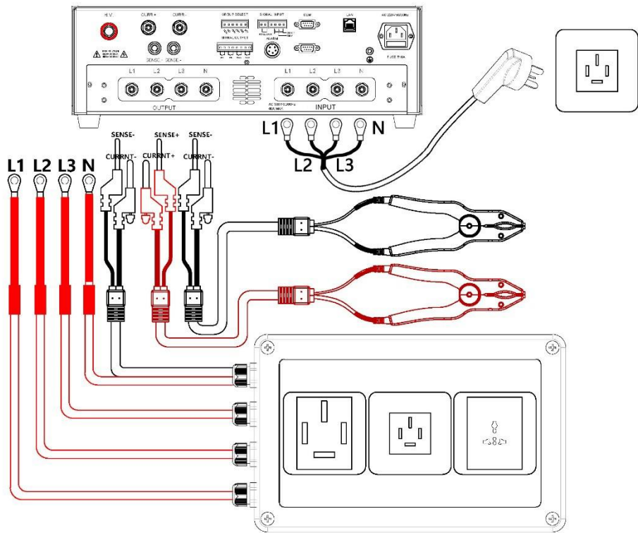
图 5-1-2 HEX430S 连接测试盒和接地测试钳示意图
