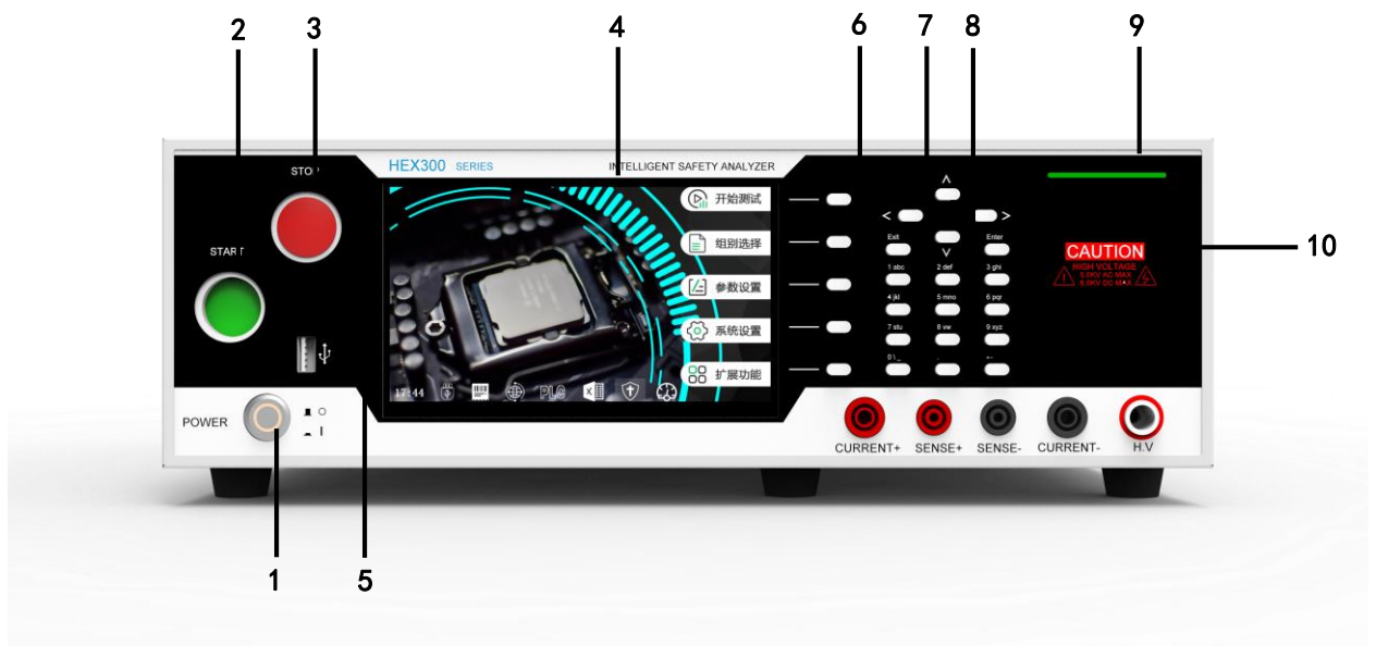
图 4-2-1 HEX300 系列前面板说明
