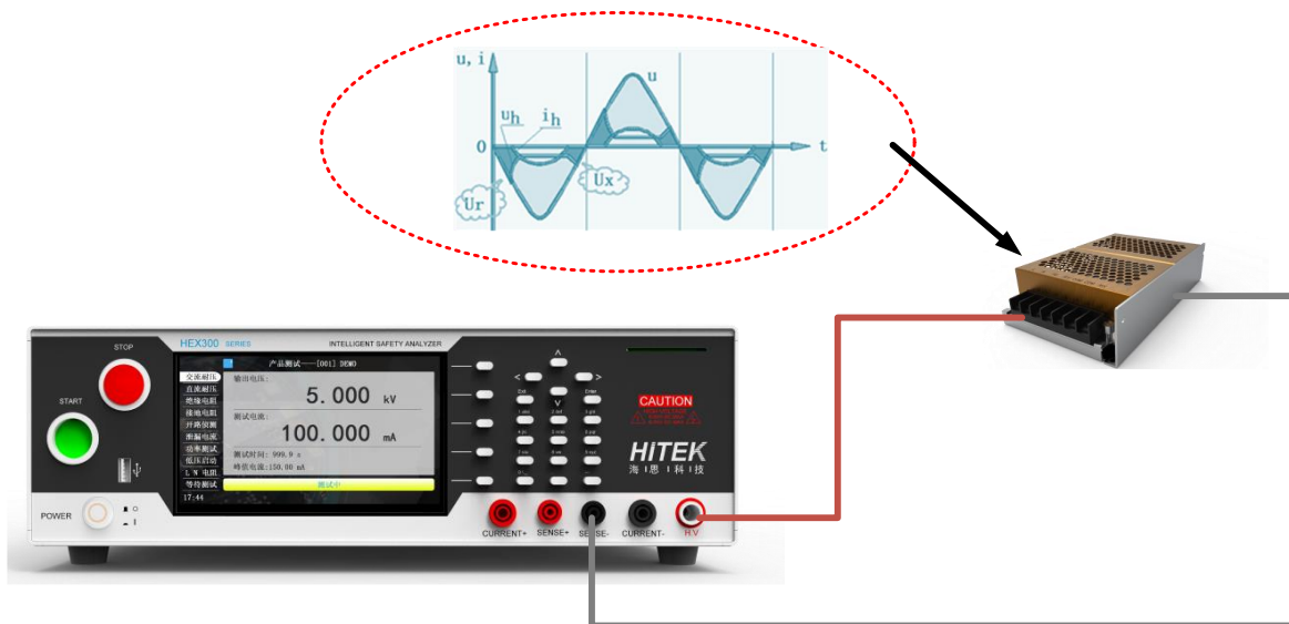
图 3-1-5 电弧侦测
