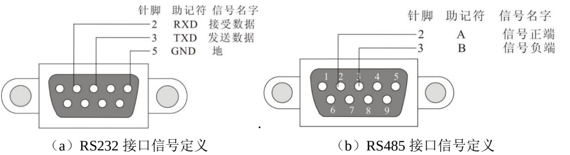
图 6-7-1 通信接口定义
