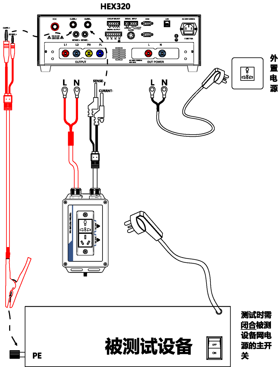
图 5-1-1 连接测试盒和接地测试钳示意图
