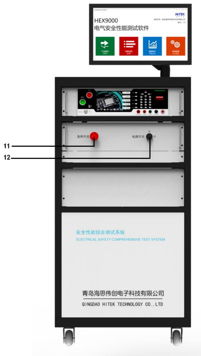
图 4-2-2 HEX430S 前面板图
