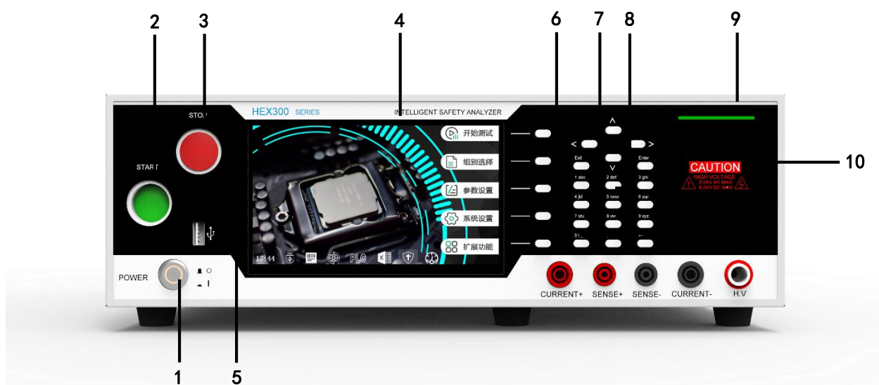
图 4-2-3 HEX410/HEX420/HEX430 前面板放大图
