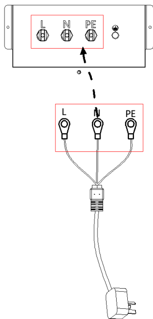
图 5-1-3 HEX410/HEX420 连接本机电源
