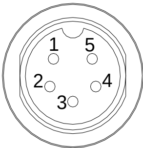
图 6-1-1 报警灯口插座（公）
