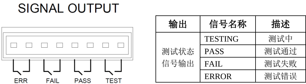
图 6-2-1 PLC 接口插座（公）
