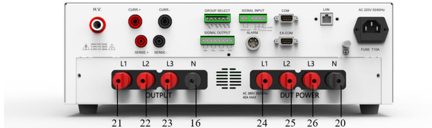
HEX330 后面板
