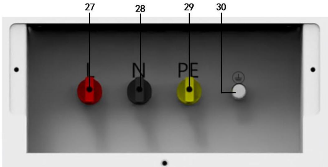
图 4-3-5 HEX410S/HEX420S 系列后面板放大图 2
