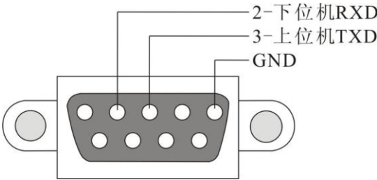
图 8-2-1 通信接口
