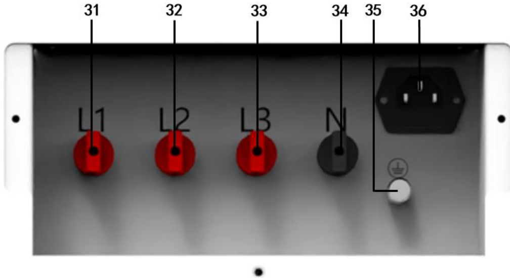
图 4-3-6 HEX430S 系列后面板放大图 3
