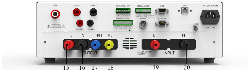
HEX320 后面板
