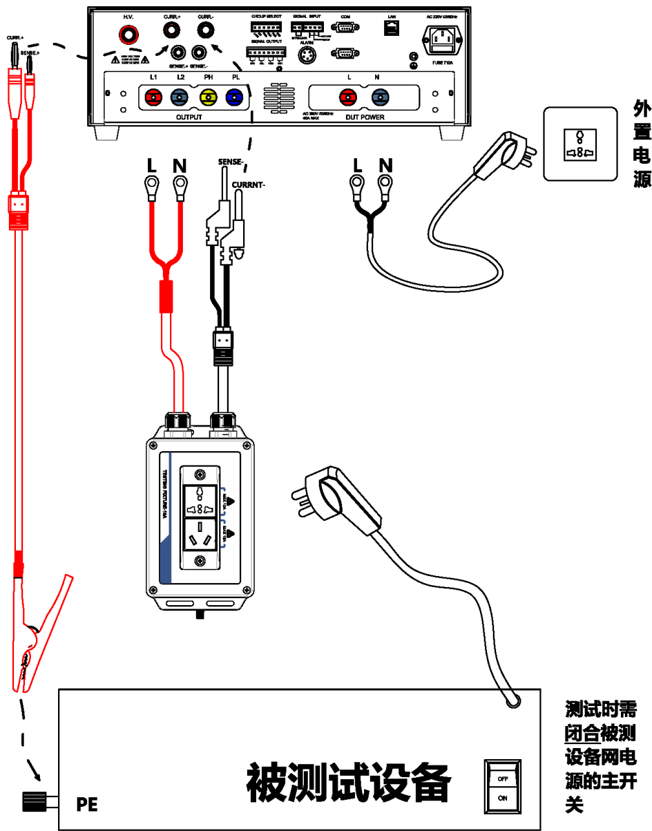
图 5-1-1HEX410S/HEX420S 连接测试盒和接地测试钳示意图
