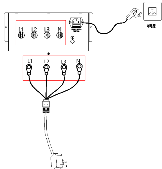
图 5-1-4 HEX430 连接本机电源
