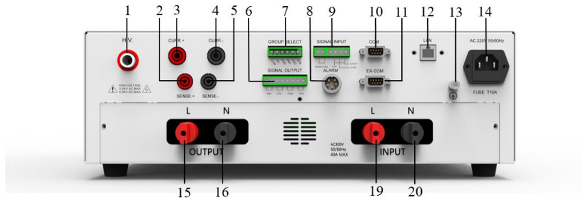
HEX310 后面板
