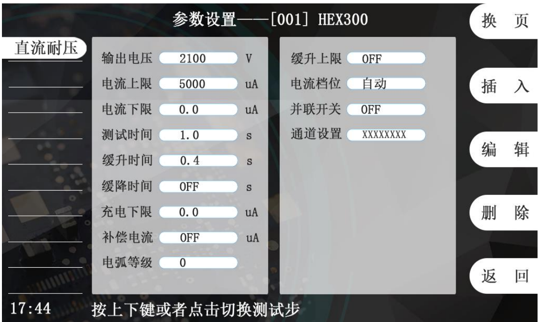
图 5-5-3 直流耐压设置界面
