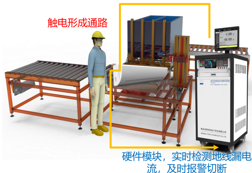
图 3-1-1 漏电快速断电保护原理
