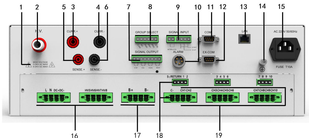
图 4-2-4 HEX450 系列后面板放大图
