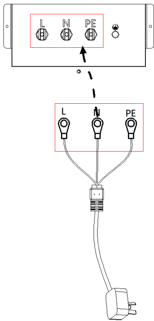
图 5-1-2 连接本机电源
