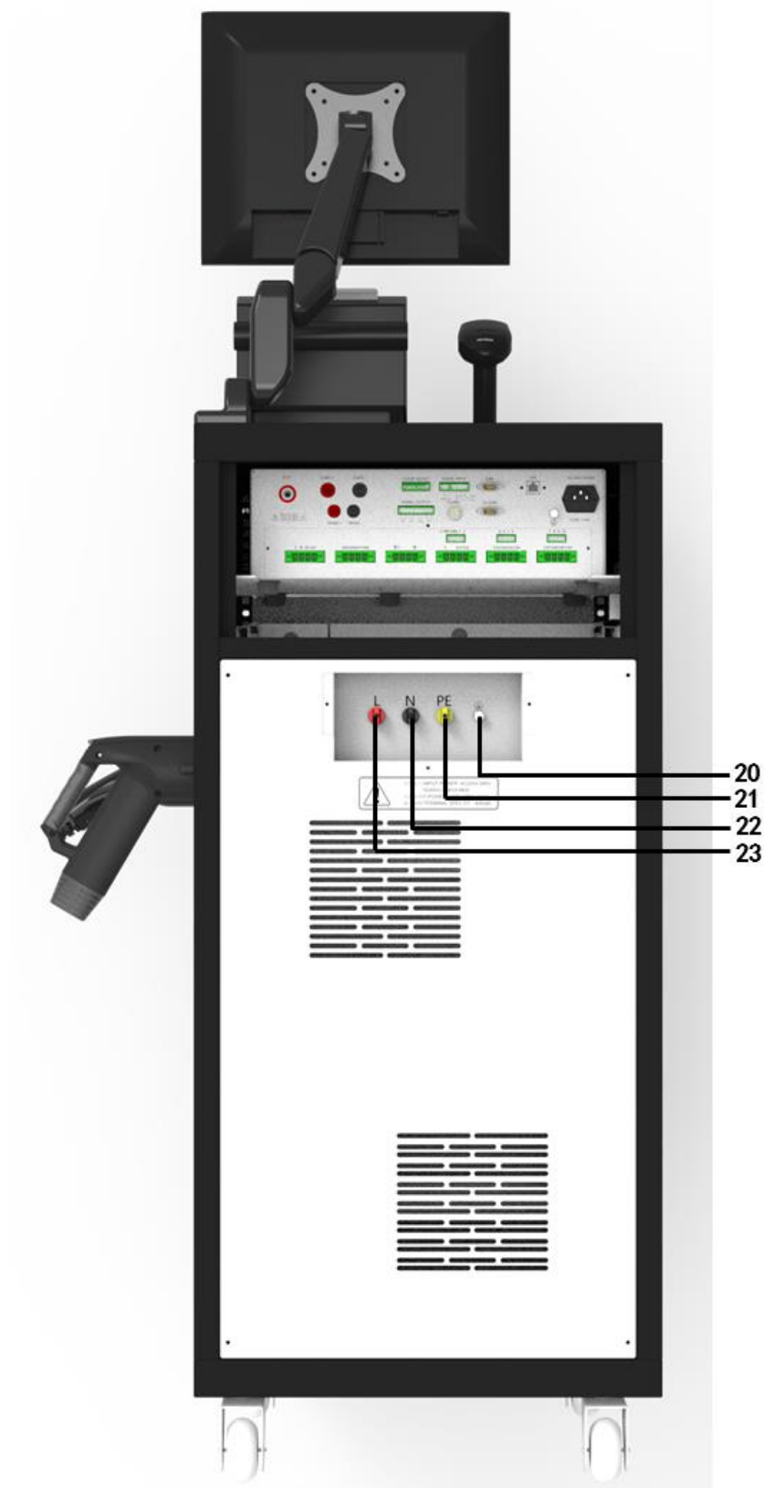
图 4-2-3 HEX450 系列后面板图
